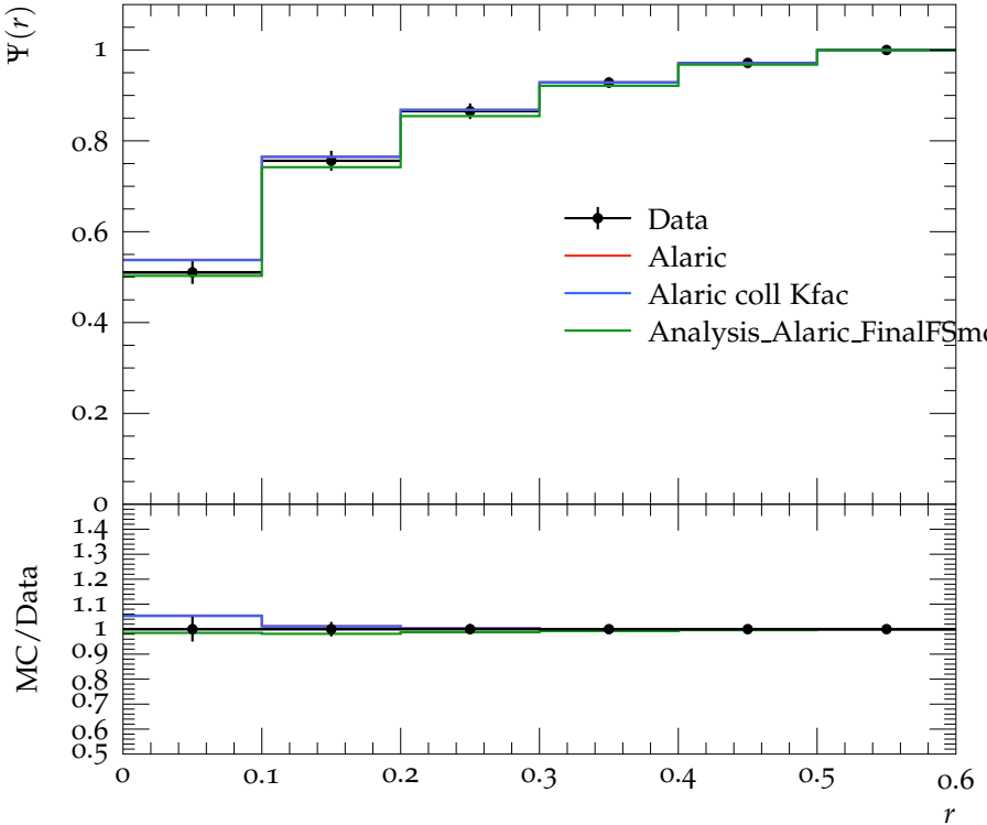
Jet shape \Psi for p_{\perp} \in 60\text{--}80\text{ GeV} , y \in 0.8\text{--}1.2
