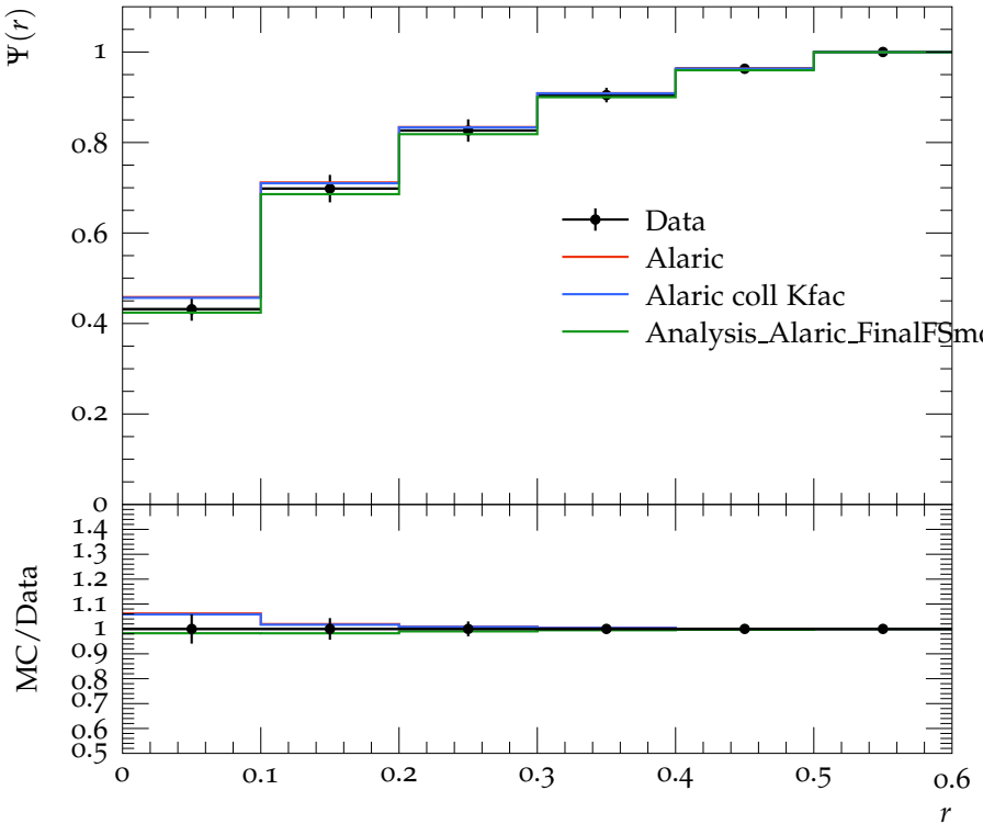
Jet shape \Psi for p_{\perp} \in 40\text{--}60\text{ GeV} , y \in 0.8\text{--}1.2
