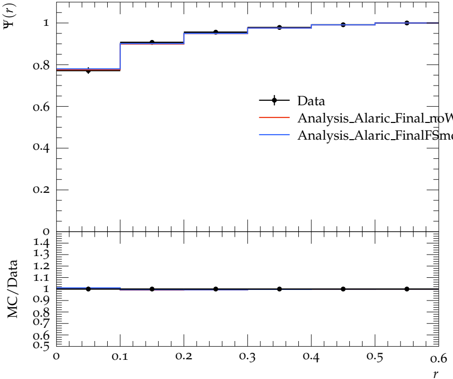
Jet shape \Psi for p_{\perp} \in 400\text{--}500\text{ GeV} , y \in 0.0\text{--}2.8
