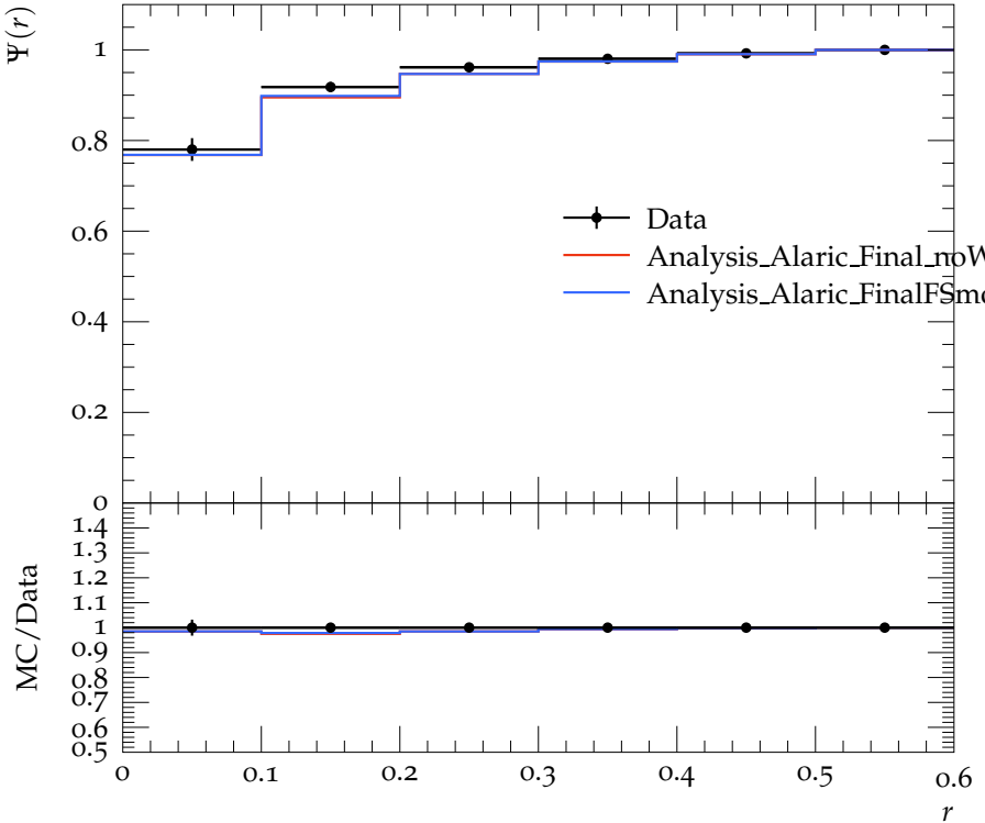
Jet shape \Psi for p_{\perp} \in 400\text{--}500\text{ GeV} , y \in 0.3\text{--}0.8
