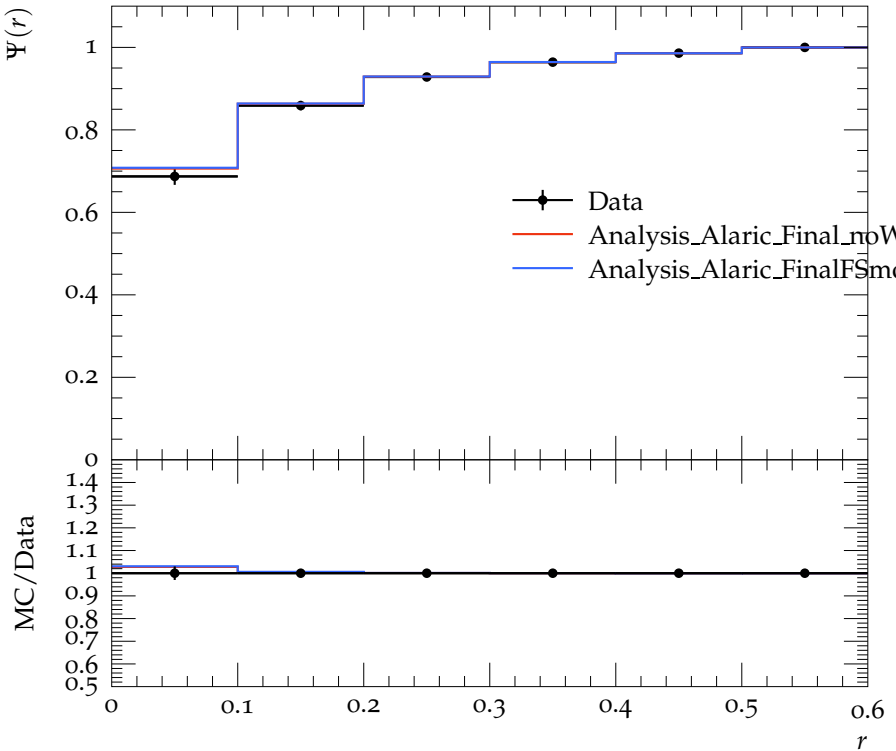
Jet shape \Psi for p_{\perp} \in 210\text{--}260\text{ GeV} , y \in 0.3\text{--}0.8
