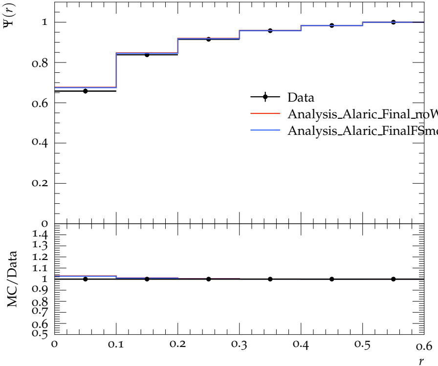
Jet shape \Psi for p_{\perp} \in 160\text{--}210\text{ GeV} , y \in 0.3\text{--}0.8
