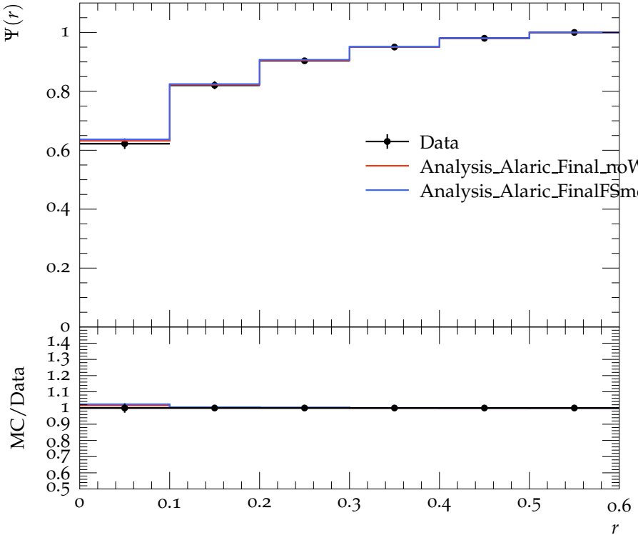
Jet shape \Psi for p_{\perp} \in 110\text{--}160\text{ GeV} , y \in 0.3\text{--}0.8
