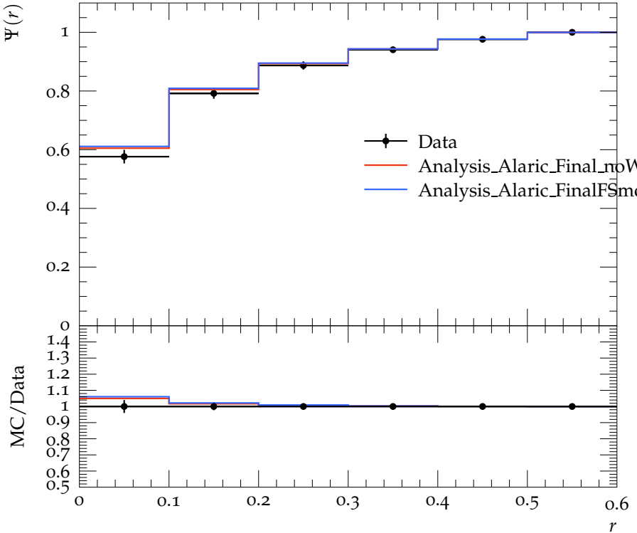
Jet shape \Psi for p_{\perp} \in 80\text{--}110\text{ GeV} , y \in 1.2\text{--}2.1
