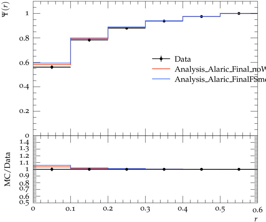
Jet shape \Psi for p_{\perp} \in 80\text{--}110\text{ GeV} , y \in 0.0\text{--}0.3
