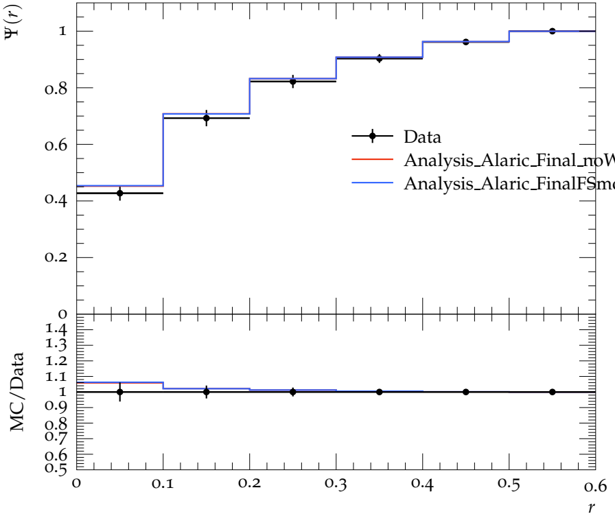
Jet shape \Psi for p_{\perp} \in 40\text{--}60\text{ GeV} , y \in 0.3\text{--}0.8
