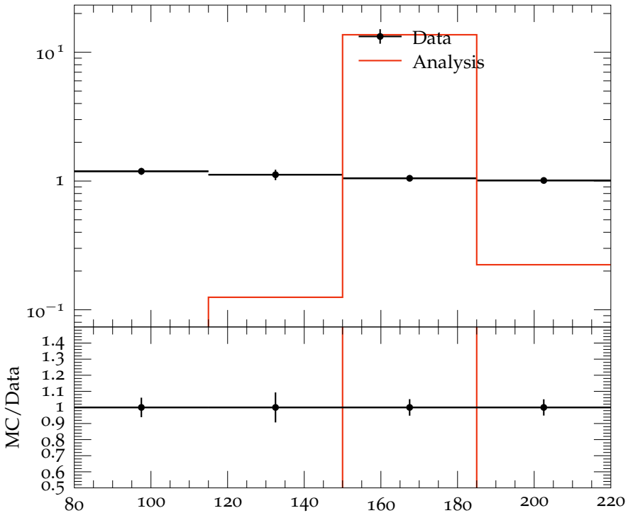
R_2 vs W , 4 < \eta < 5
