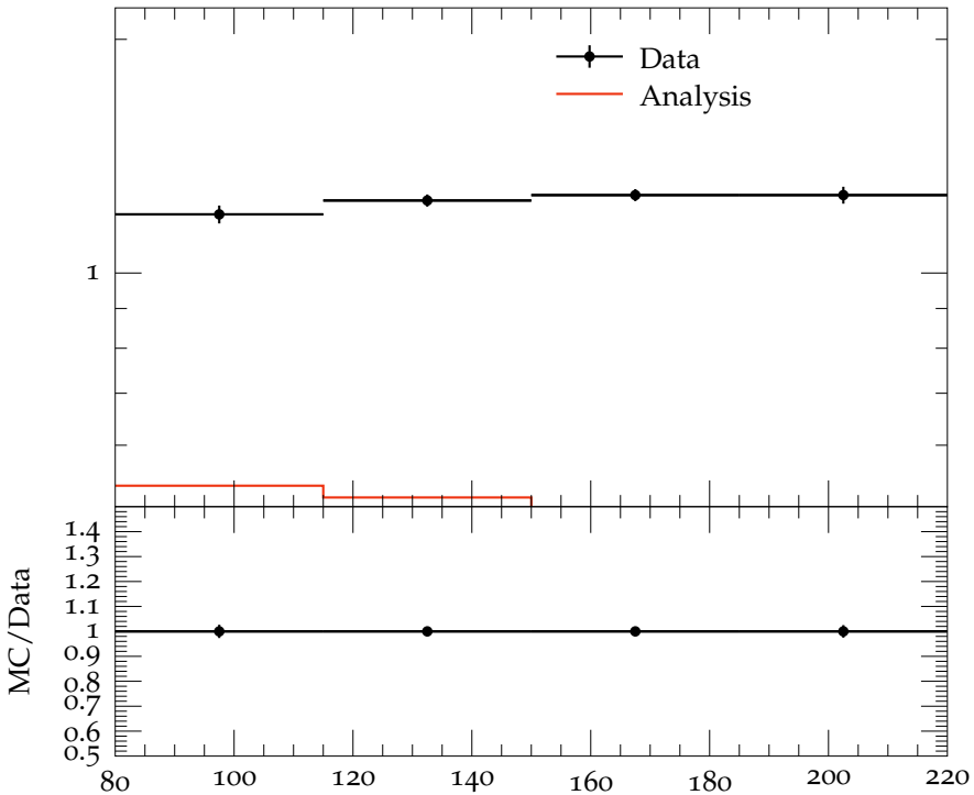
R_2 vs W , 1 < \eta < 3
