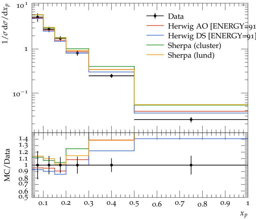
\omega(782) spectrum
