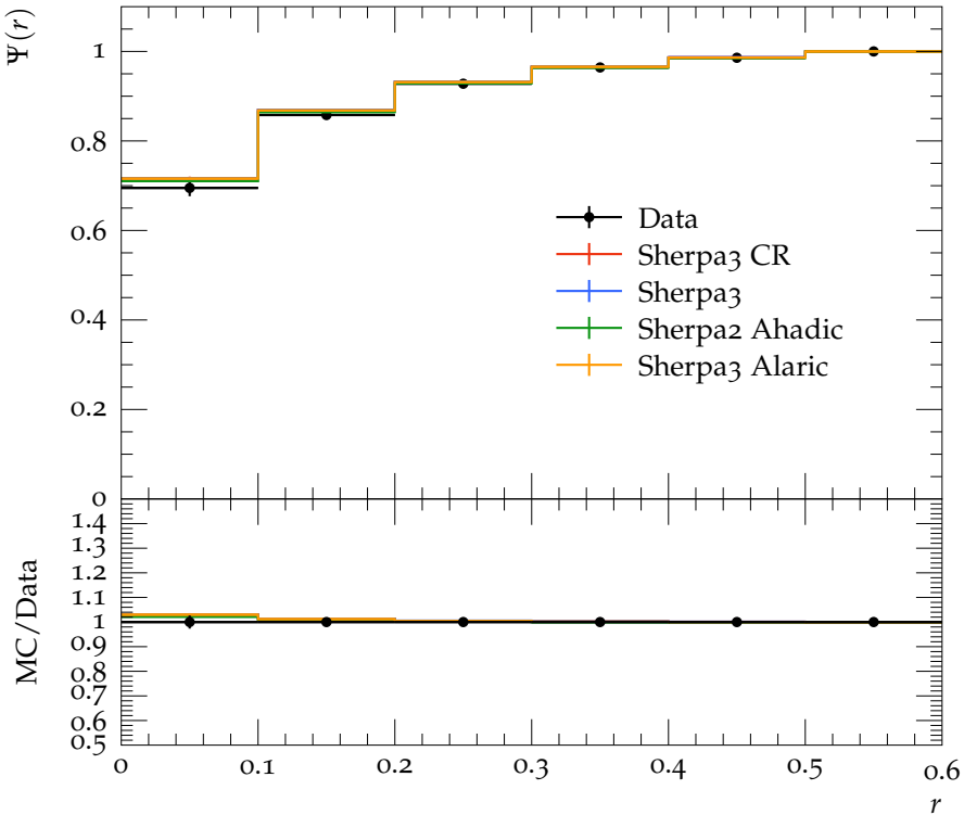
Jet shape \Psi for p_{\perp} \in 210\text{--}260\text{ GeV} , y \in 0.8\text{--}1.2
