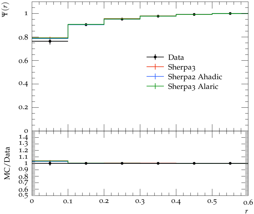
Jet shape \Psi for p_{\perp} \in 500\text{--}600\text{ GeV} , y \in 0.0\text{--}2.8
