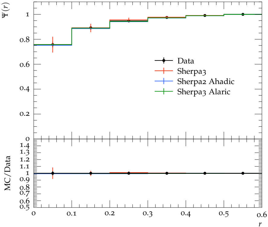
Jet shape \Psi for p_{\perp} \in 310\text{--}400\text{ GeV} , y \in 0.8\text{--}1.2
