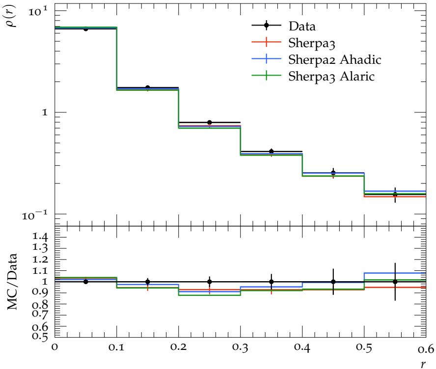
Jet shape \rho for p_{\perp} \in 160\text{--}210\text{ GeV} , y \in 0.8\text{--}1.2
