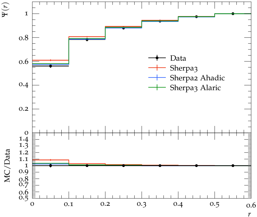
Jet shape \Psi for p_{\perp} \in 80\text{--}110\text{ GeV} , y \in 0.0\text{--}0.3
