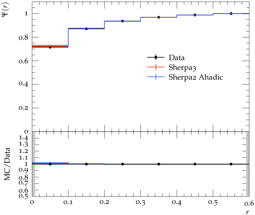
Jet shape \Psi for p_{\perp} \in 260\text{--}310\text{ GeV} , y \in 0.8\text{--}1.2
