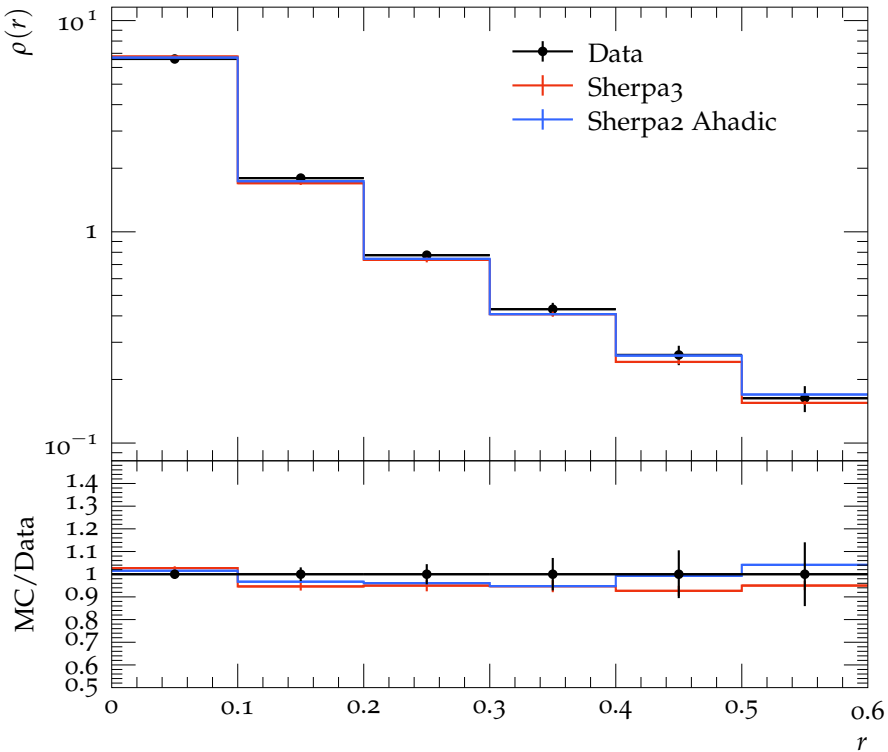
Jet shape \rho for p_{\perp} \in 160\text{--}210\text{ GeV} , y \in 0.3\text{--}0.8
