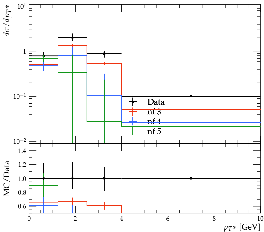
Transverse D* momentum HCM
