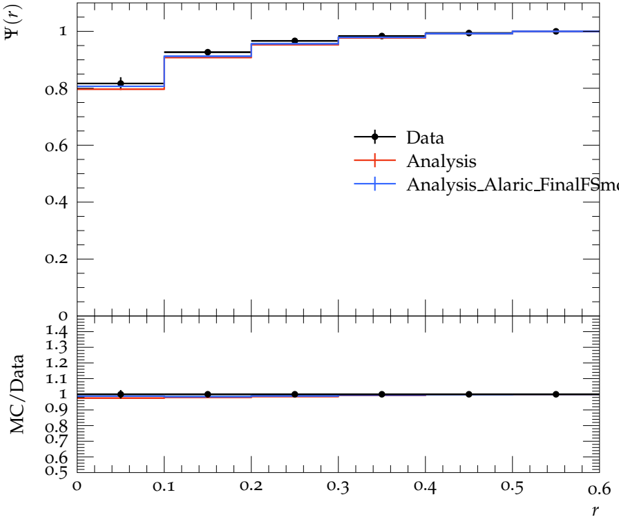
Jet shape \Psi for p_{\perp} \in 400\text{--}500\text{ GeV} , y \in 1.2\text{--}2.1
