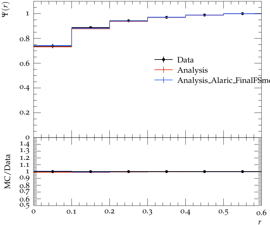
Jet shape \Psi for p_{\perp} \in 310\text{--}400\text{ GeV} , y \in 0.0\text{--}0.3
