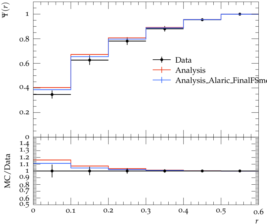
Jet shape \Psi for p_{\perp} \in 30\text{--}40\text{ GeV} , y \in 0.8\text{--}1.2
