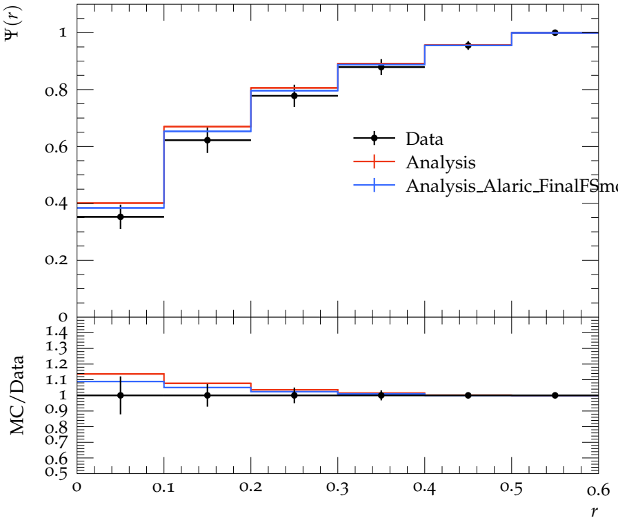
Jet shape \Psi for p_{\perp} \in 30\text{--}40\text{ GeV} , y \in 0.3\text{--}0.8
